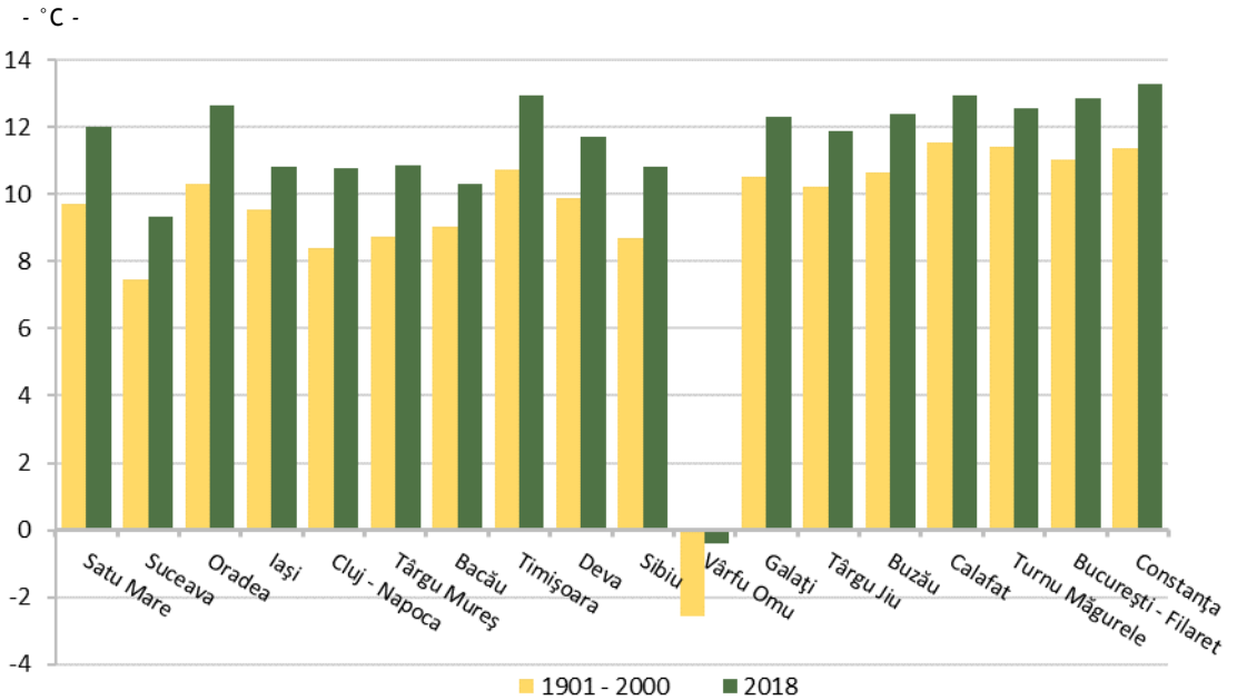
Fig. 13.2.1. Temperaturile medii anuale la nivelul României
