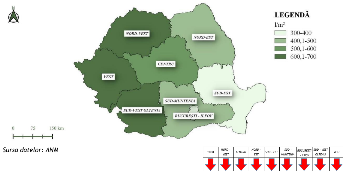
Figura M21. Cantitatea anuală de precipitații, pe regiuni de dezvoltare, în anul 2022
