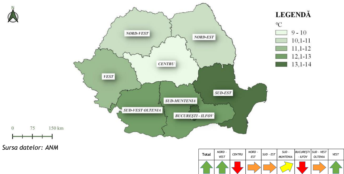
Figura M20. Temperatura medie anuală, pe regiuni de dezvoltare, în anul 2022
